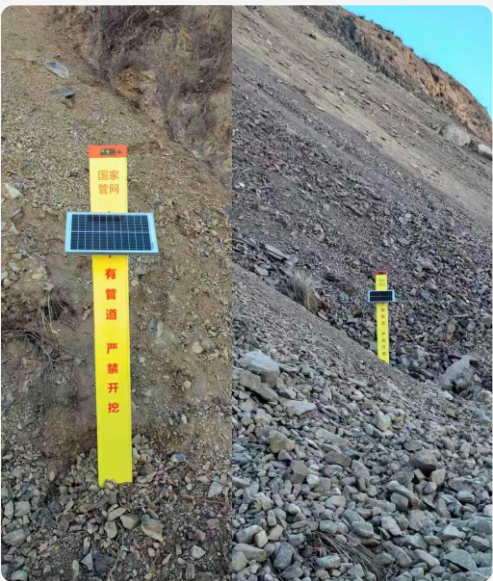
项目名称：不稳定边坡监测 项目地点：甘肃.兰州
