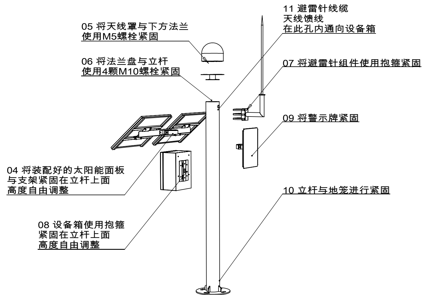
设备附件装配顺序
