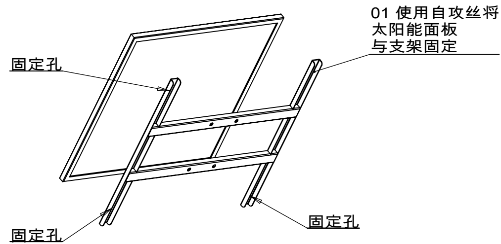
太阳能面板与支架连接
