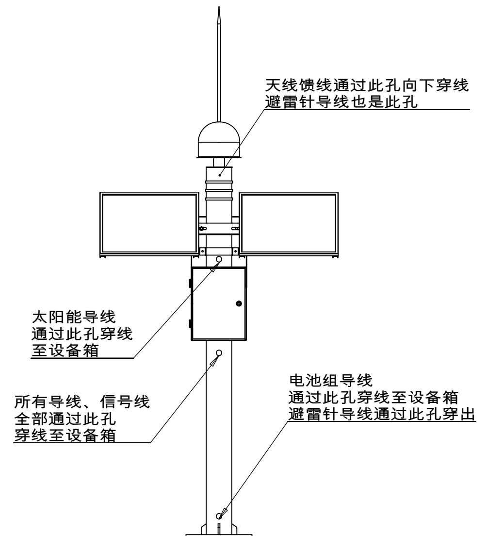
设备走线标注
