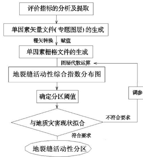
图E.1 地裂缝活动性评价流程
