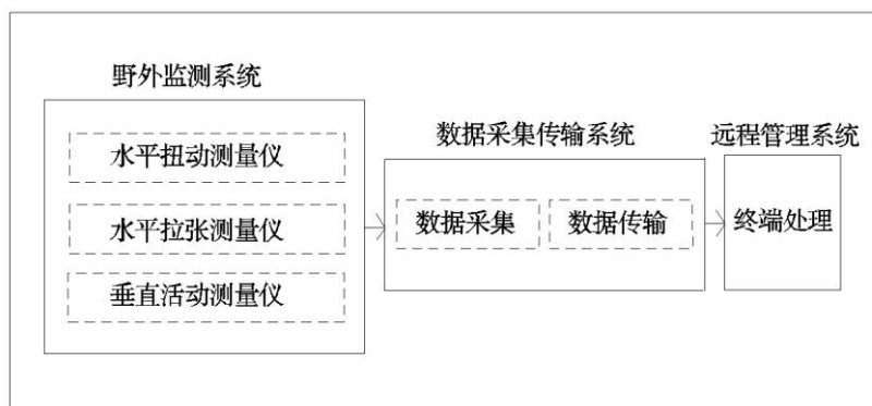
图 C.1 三维变形测量仪拓扑结构示意图
