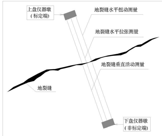
图 c. 2 三维变形测量仪平面布置示意图
