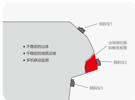
地质灾害\边坡护坡的监测应用
