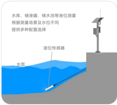
水位测量原理示意图
