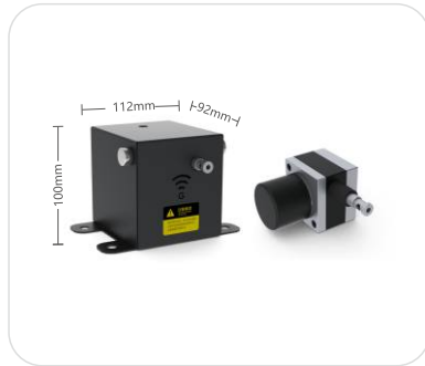
拉线位移传感器
