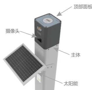
电子智慧界桩组成部分
