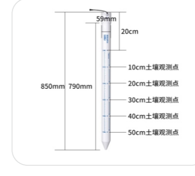
管式多层土壤水分传感器
