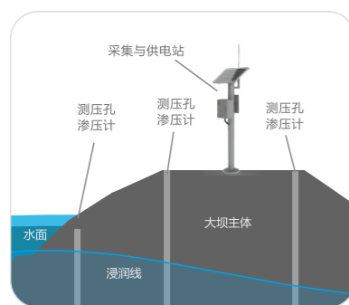
内部水压力浸润性测量示意图
