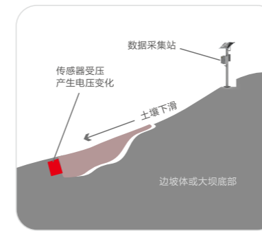
土壤压力工作示意图
