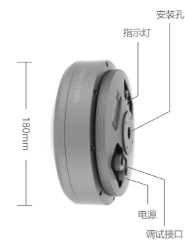
外部接口与直径尺寸
